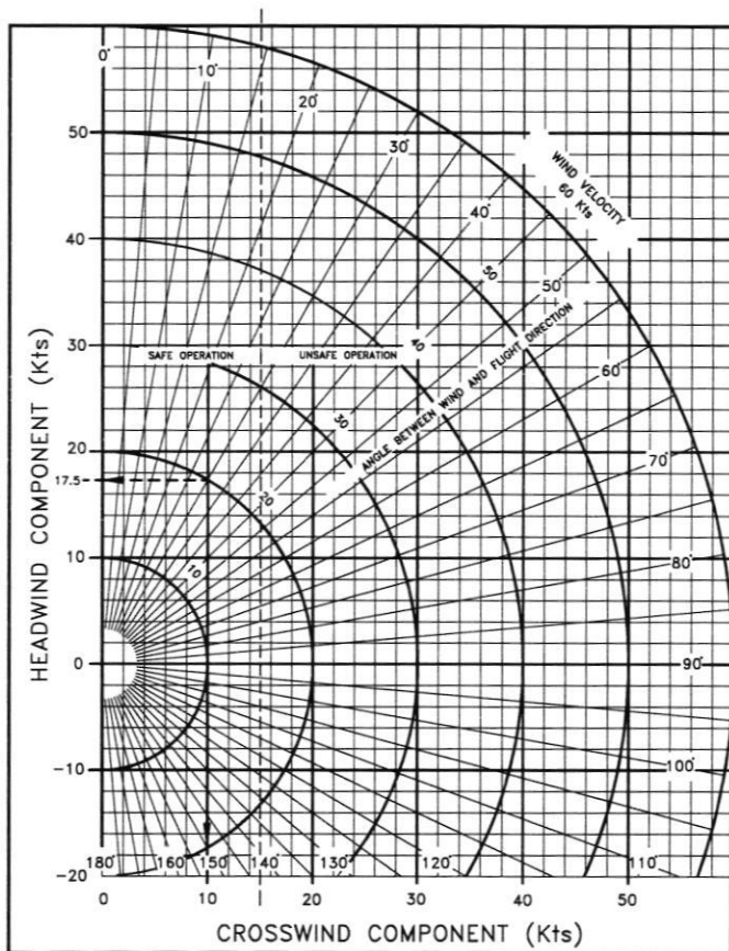
Fig. 5-3. CROSSWIND CHART
